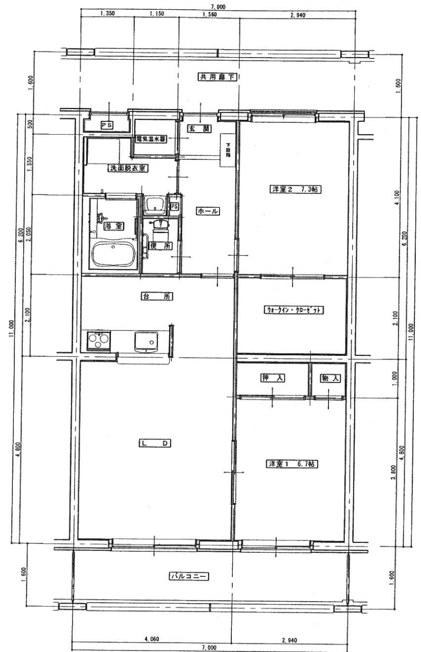
Bタイプ 2LDK平面詳細図 1/50 住戸専用面積 76.33 m 2
