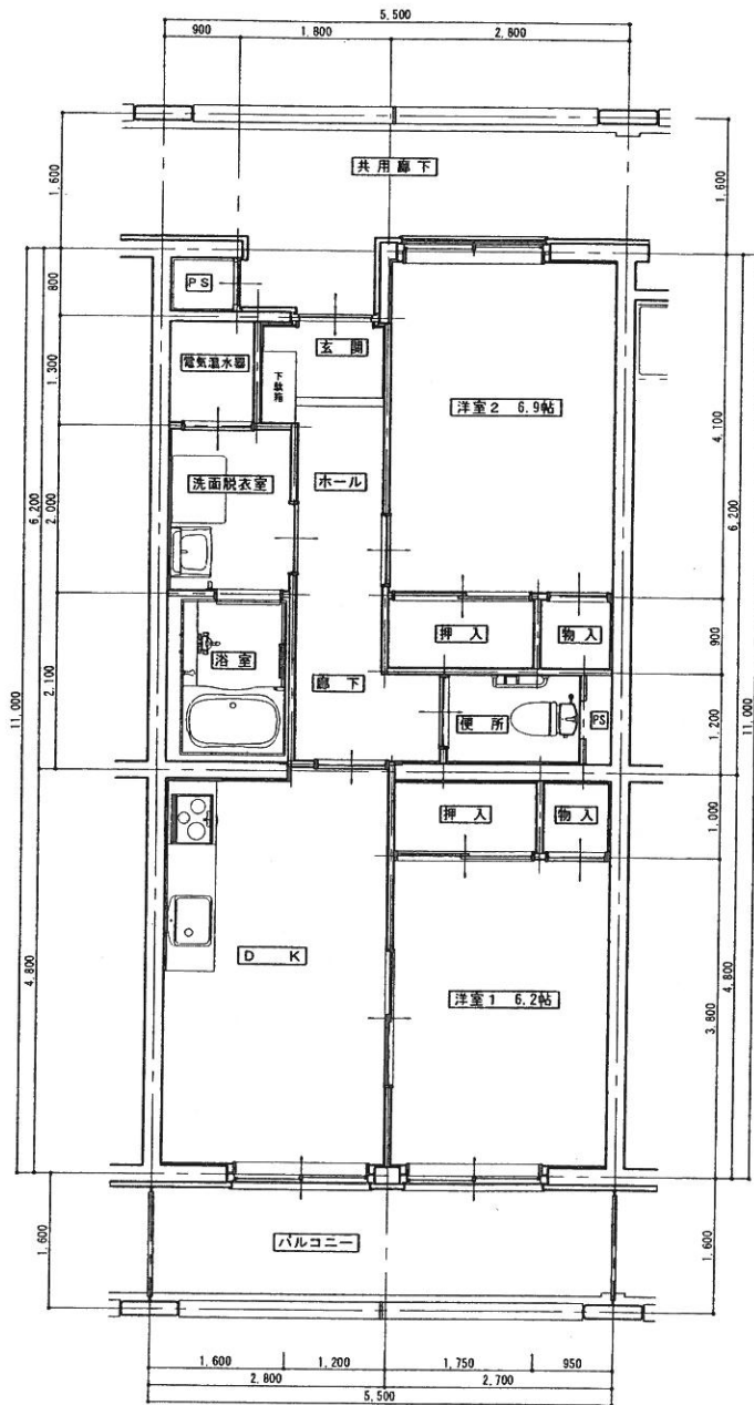
Aタイプ 2DK平面詳細図 1/50 住戸専用面積 58.34 m 2
