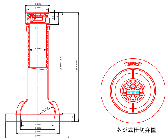
仕切弁表筐構造図（参考図）
