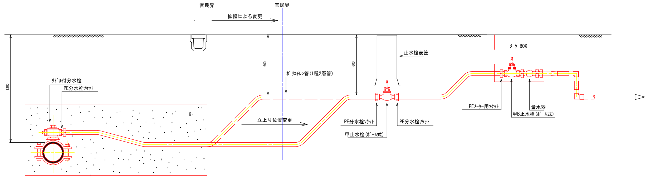
給水装置（参考図）
