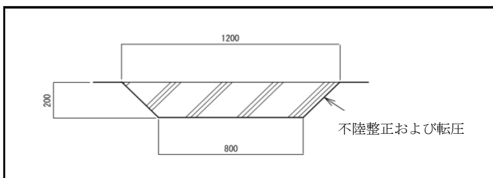
土道整備部分（断面図）
