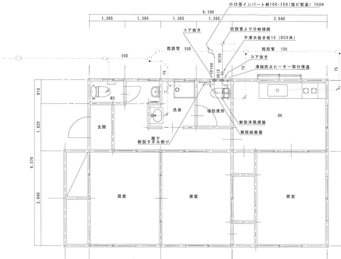
トイレ増設後平面図 S=1/50
