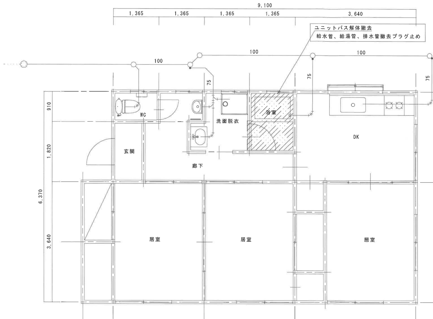
現況平面図 S=1/50
