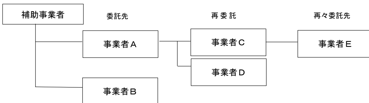
実施体制図
