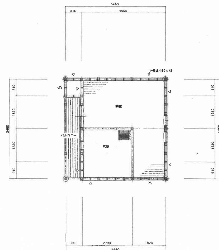
2階平面詳細図 S=1/50
