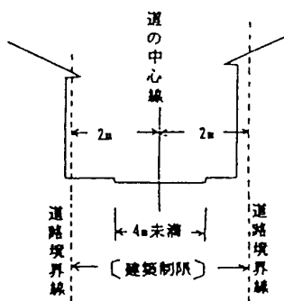
建築基準法第44条1項の場合
